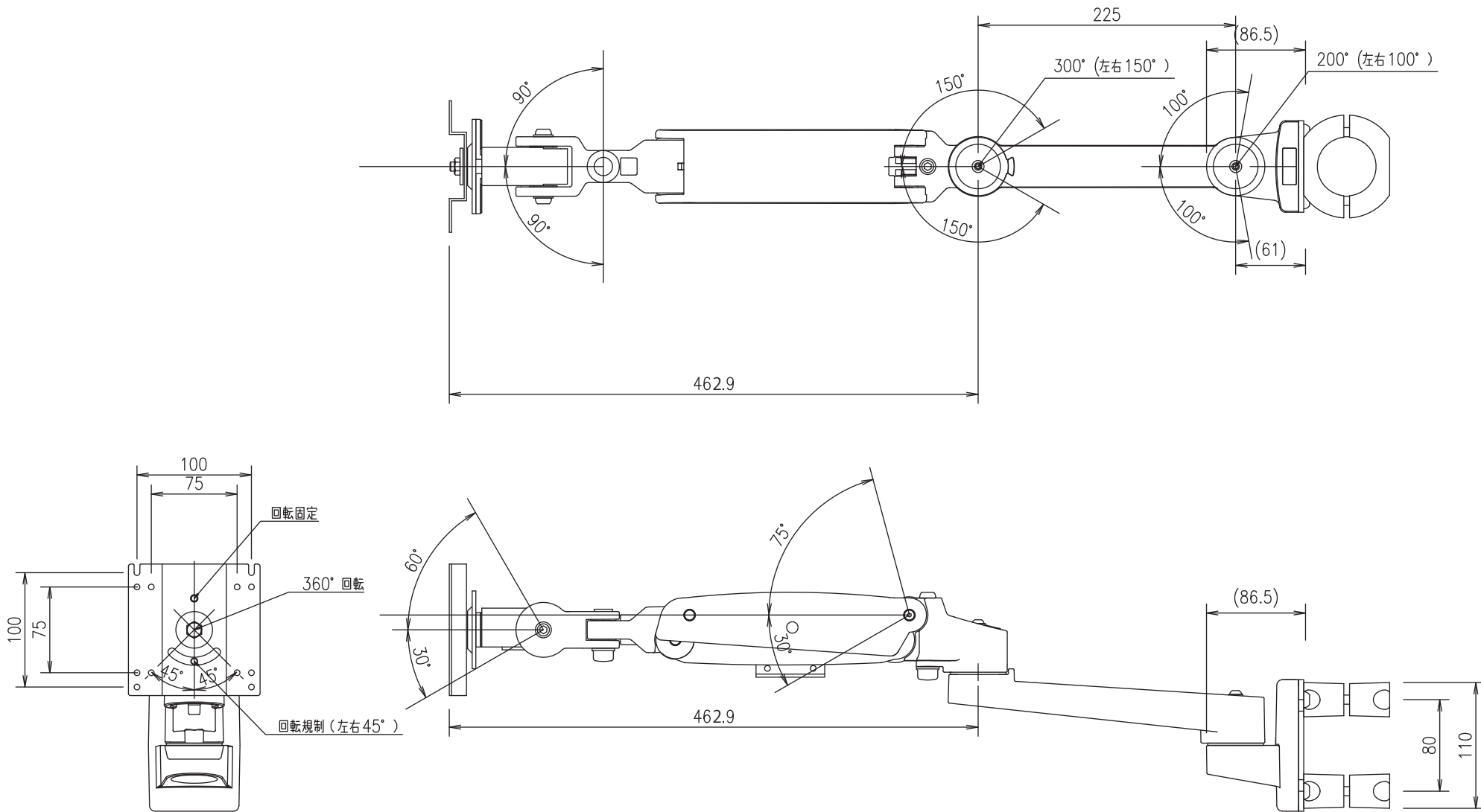
クレーンアーム本体-ボームクランプ付垂直ベース延長アーム-簡易ロック無し(型番:FFP-QA-PB-EF)
