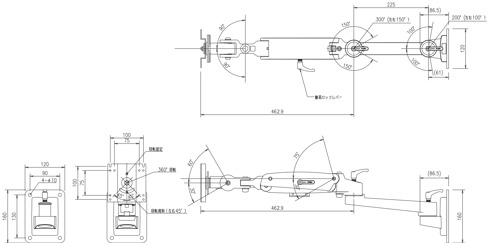
クレーンアーム-本体-直付垂直ハース-延長アーム-簡易ロック有り(型番:FFP-QAL-DBL-EFL)
