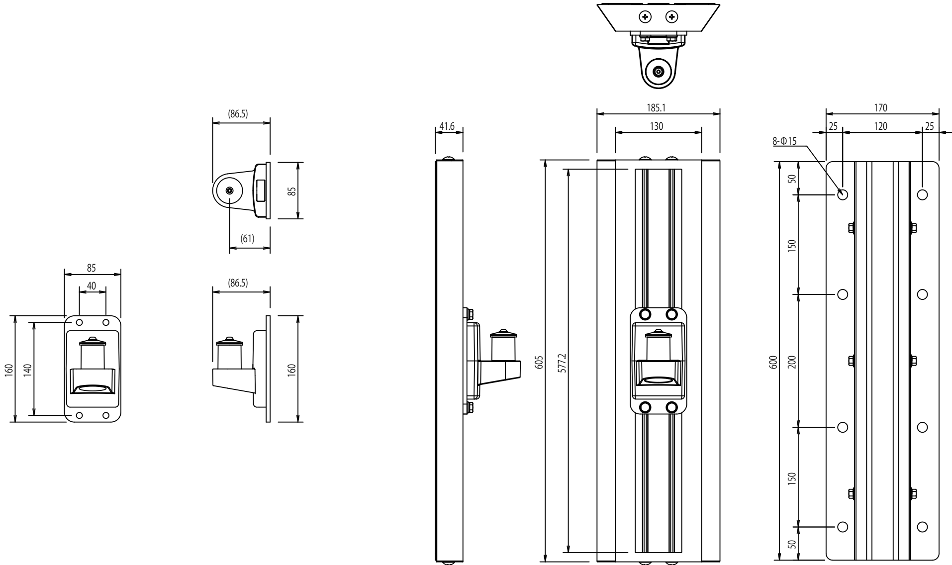
クレーンアーム縦型壁面用アルミレールレバー無し(型番:FFP-AH600)
