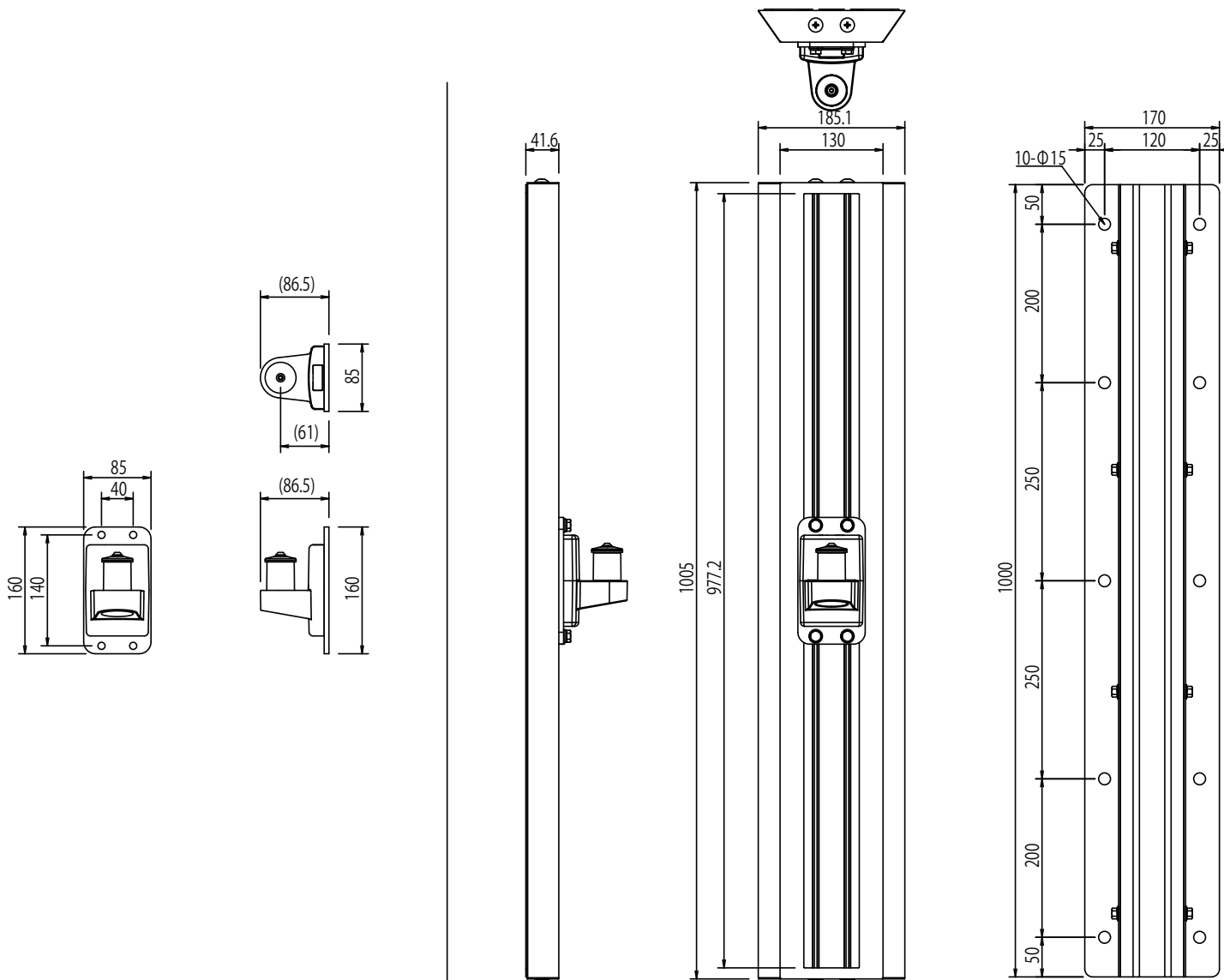
クレーンアーム縦型壁面用アルミレールレバー無し(型番:FFP-AH1000)
