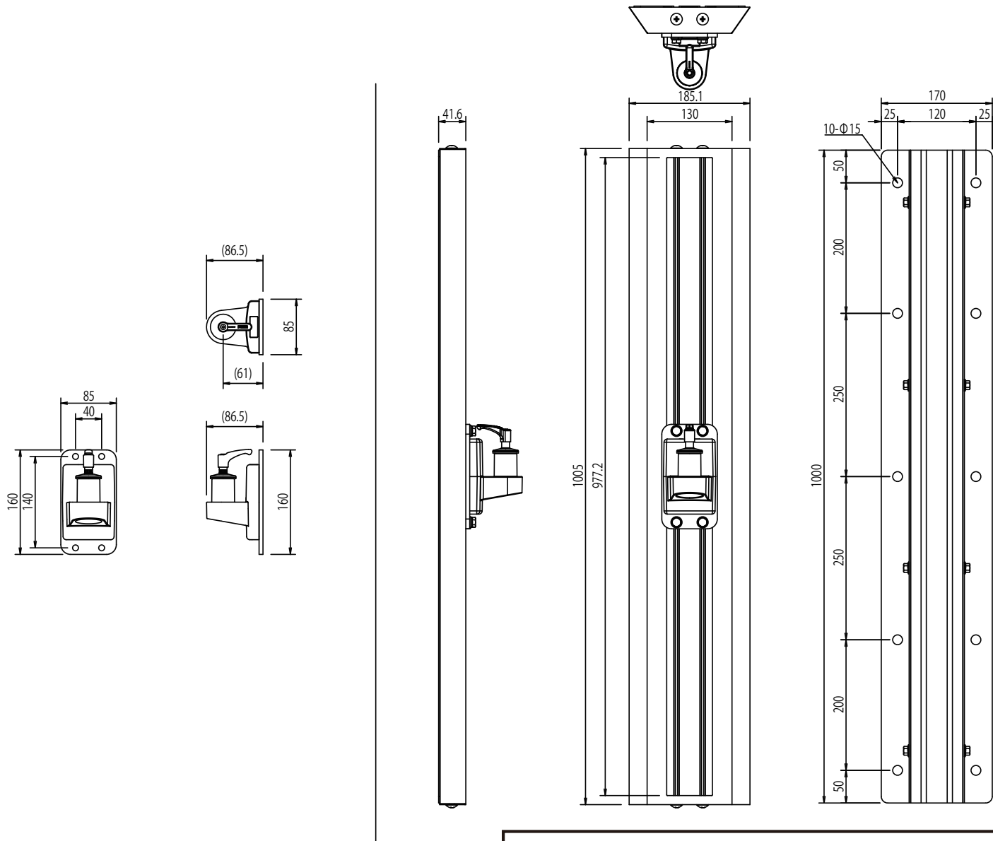
クレーンアーム縦型壁面用アルミレールレバー有り (型番:FFP-AHL1000)
