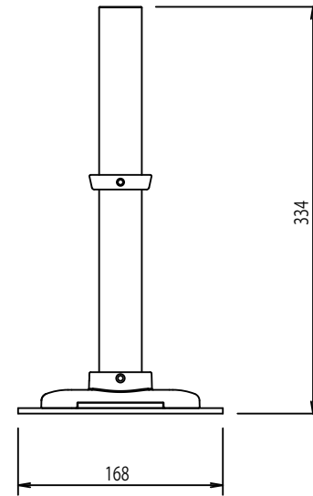
クレーンアーム直付デスクベース (型番:FFP-DDB)
