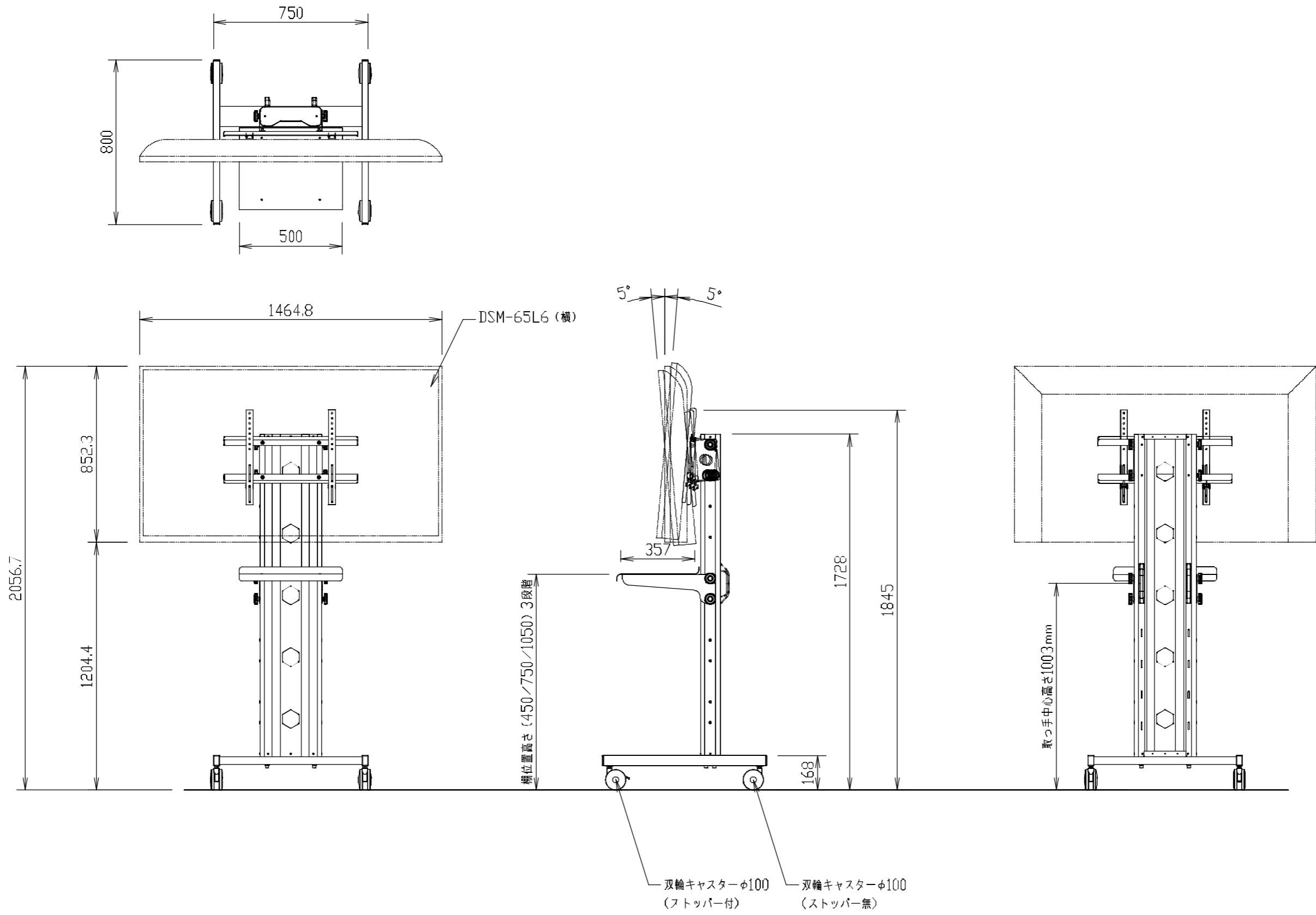
ディスプレイスタンド FTK-D-STAND50-M 外觀仕様図
