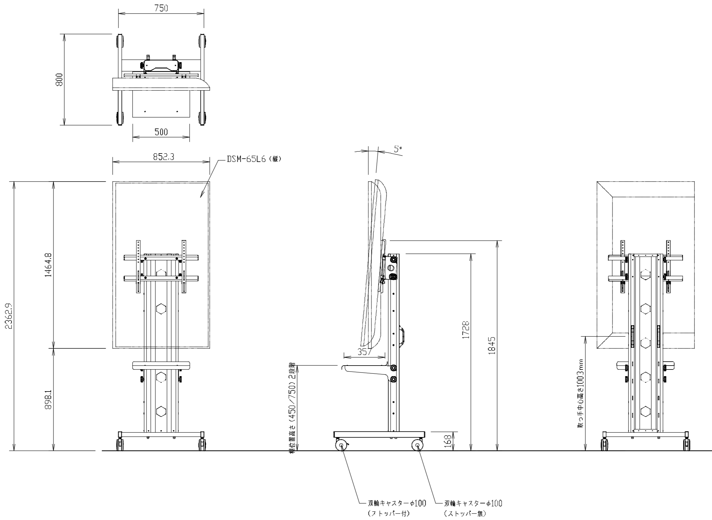
ディスプレイスタンド FTK-D-STAND50-M 外觀仕様図
