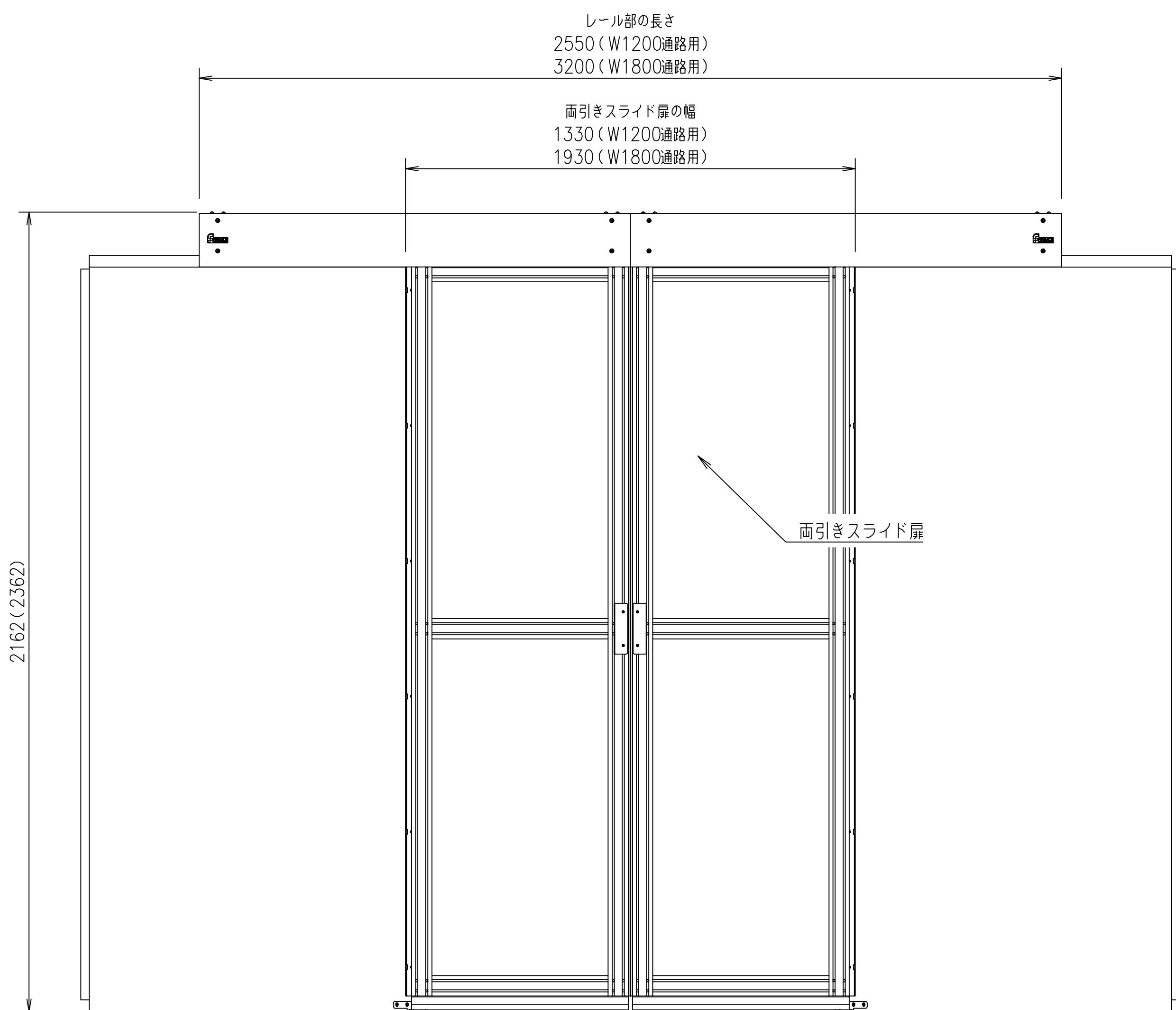
正面図 (扉が閉じている状態)
