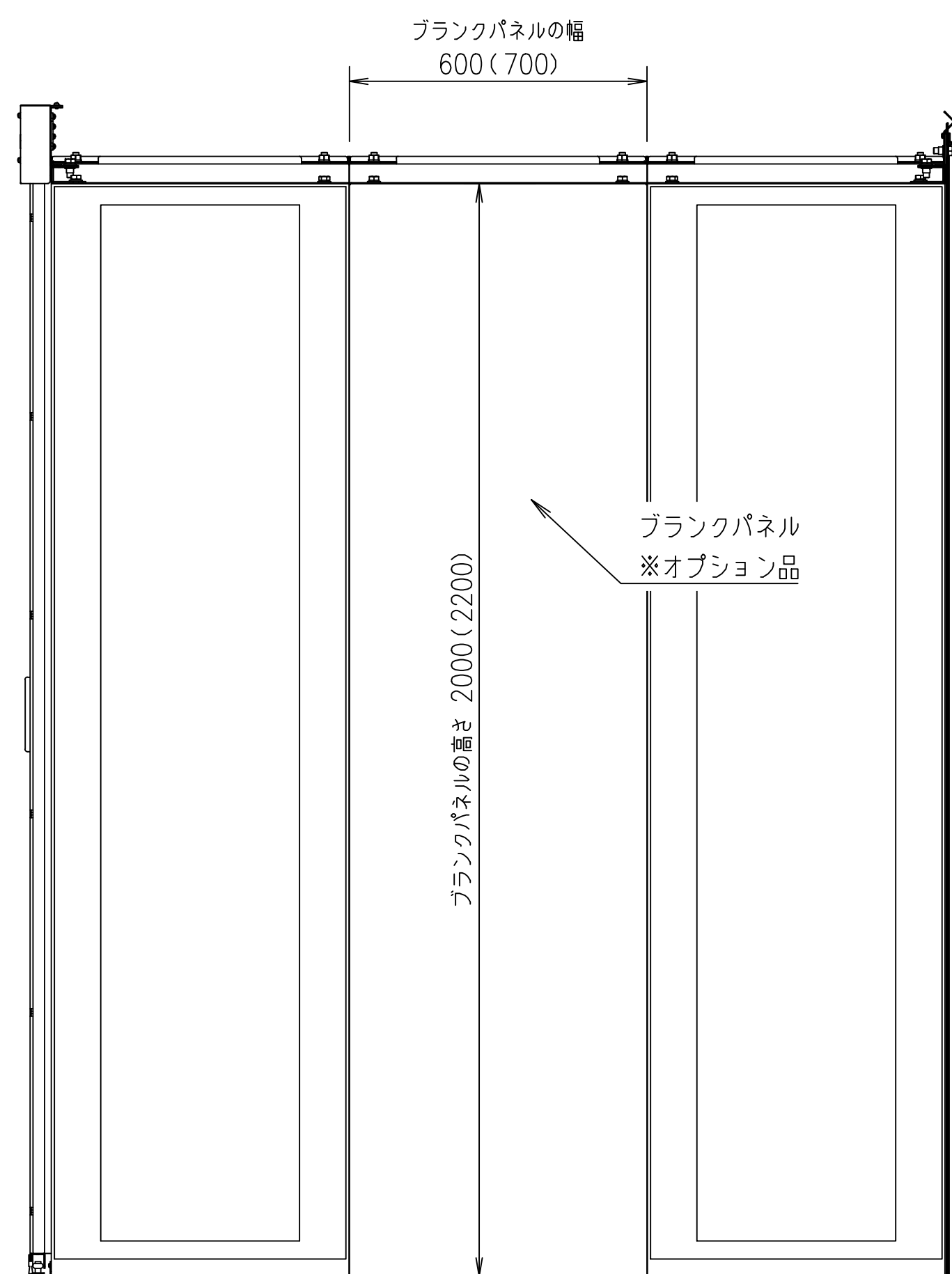
側面図
