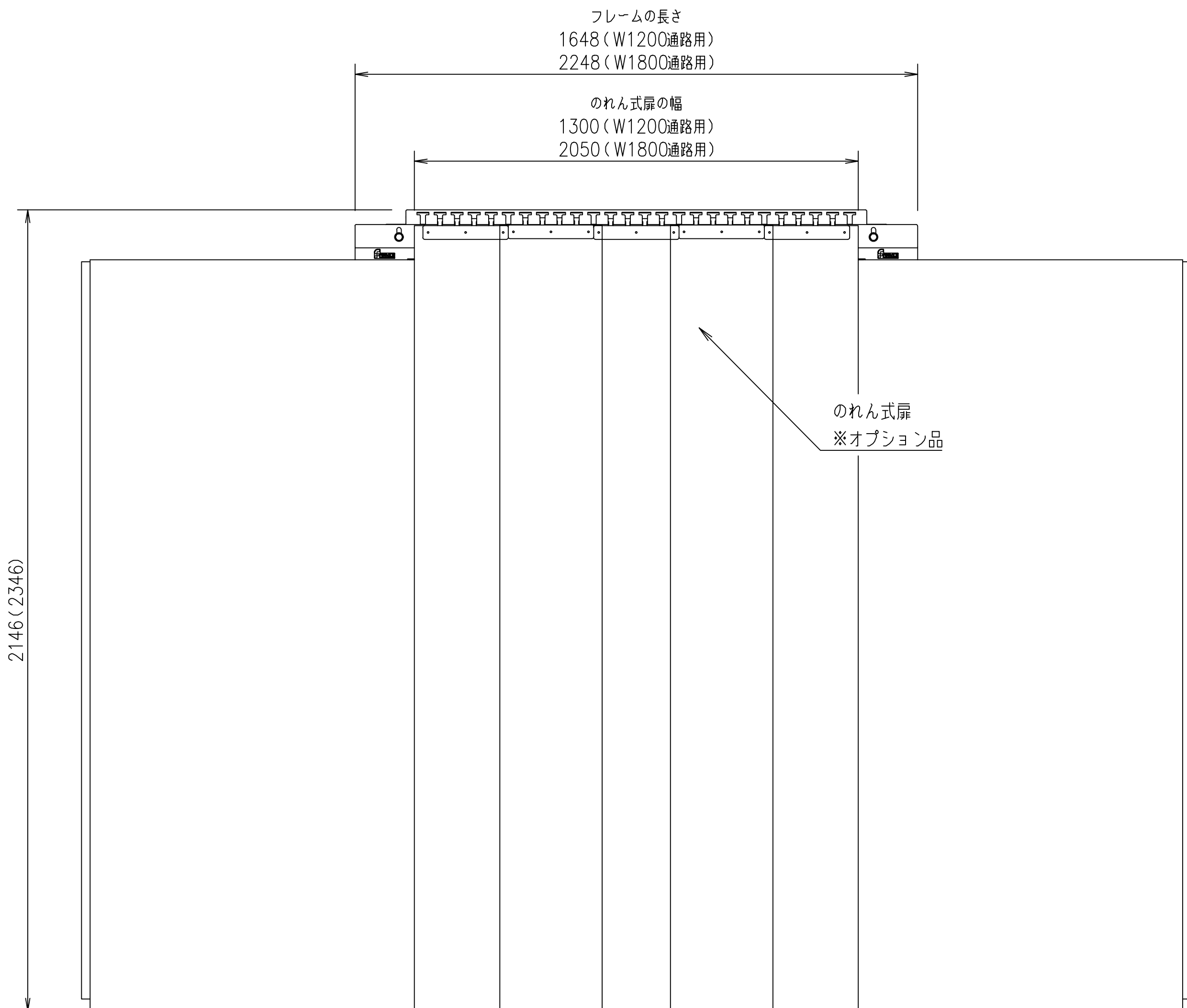
背面図
