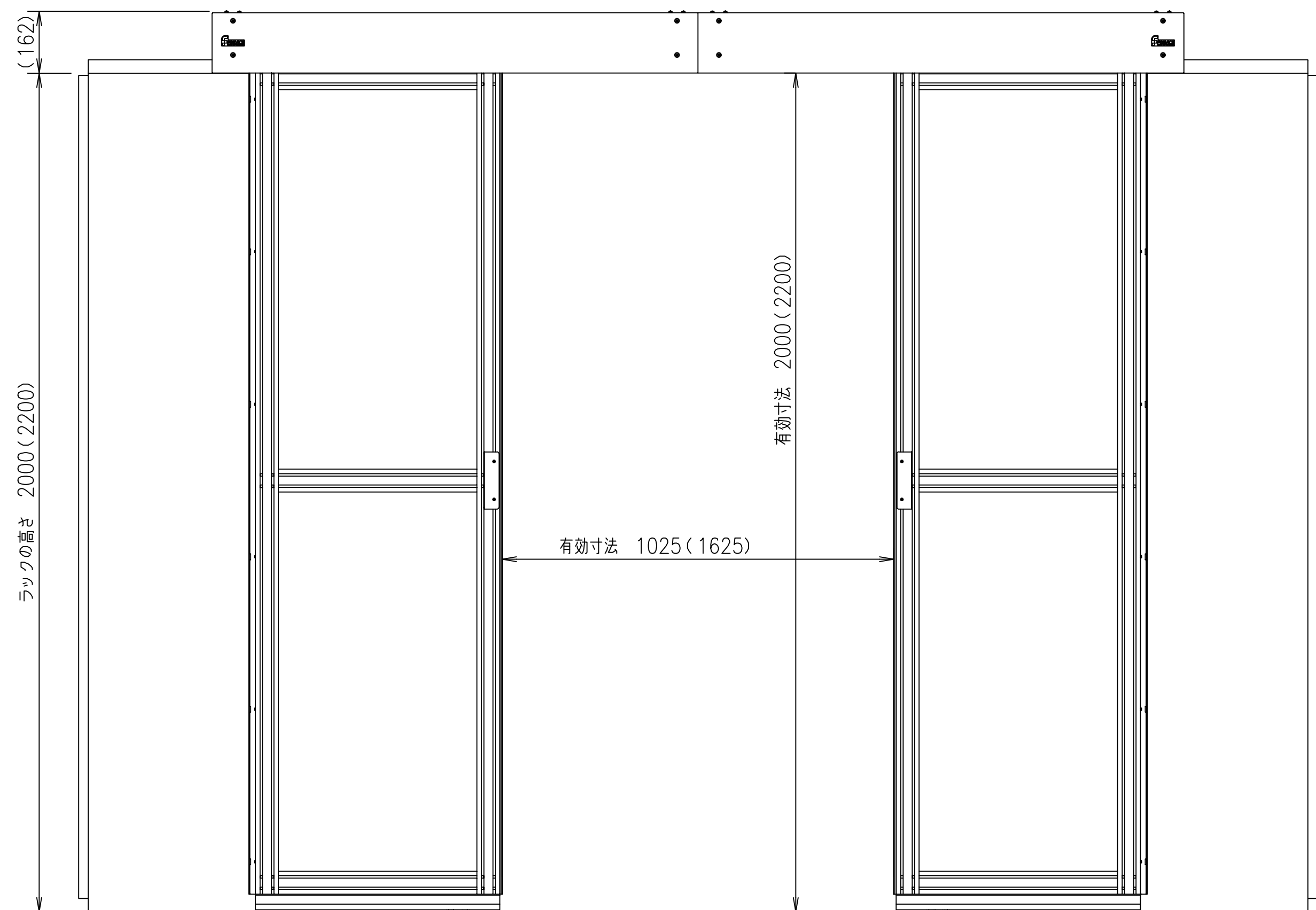
正面図 (扉が開いている状態)
