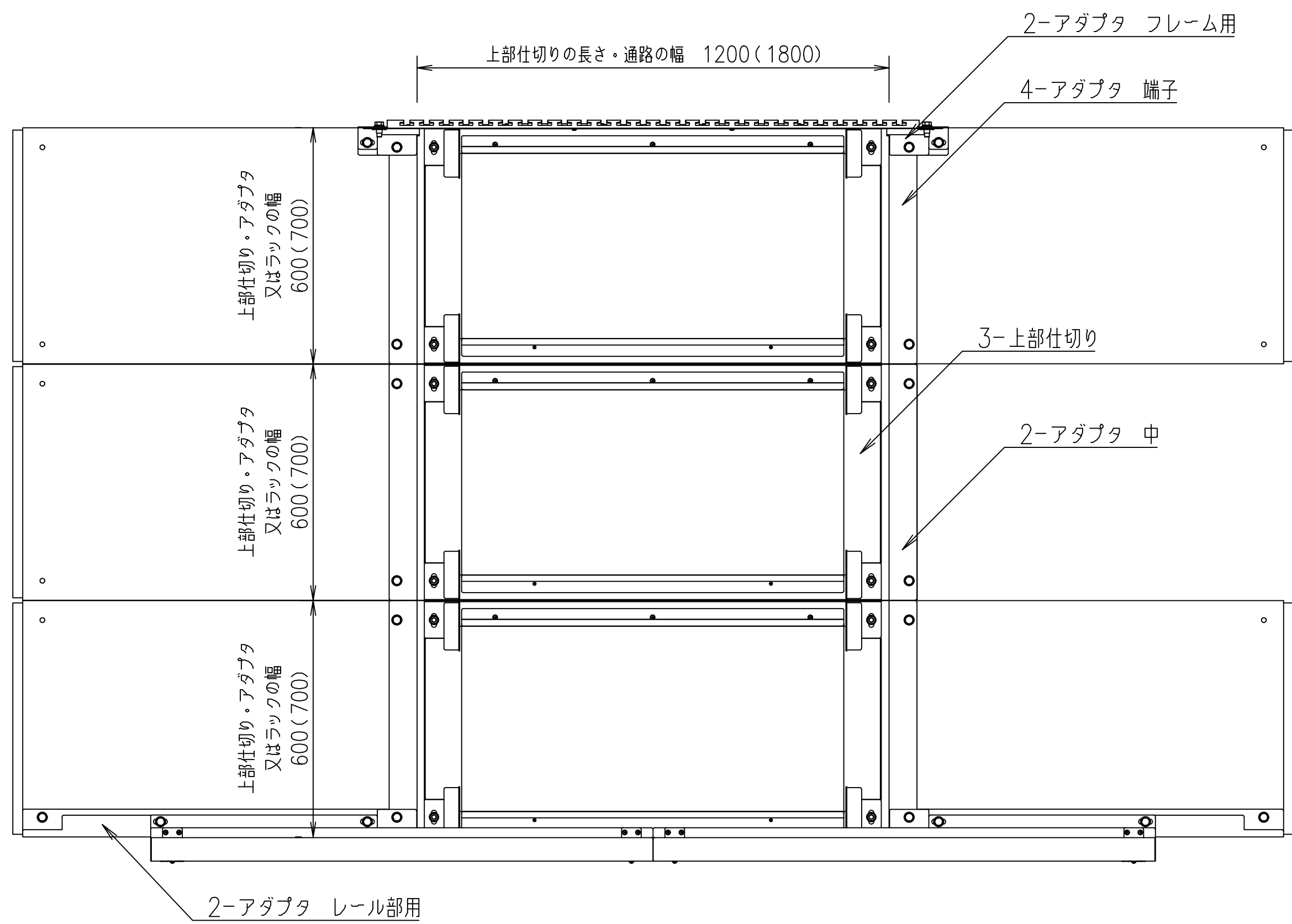
平面図
