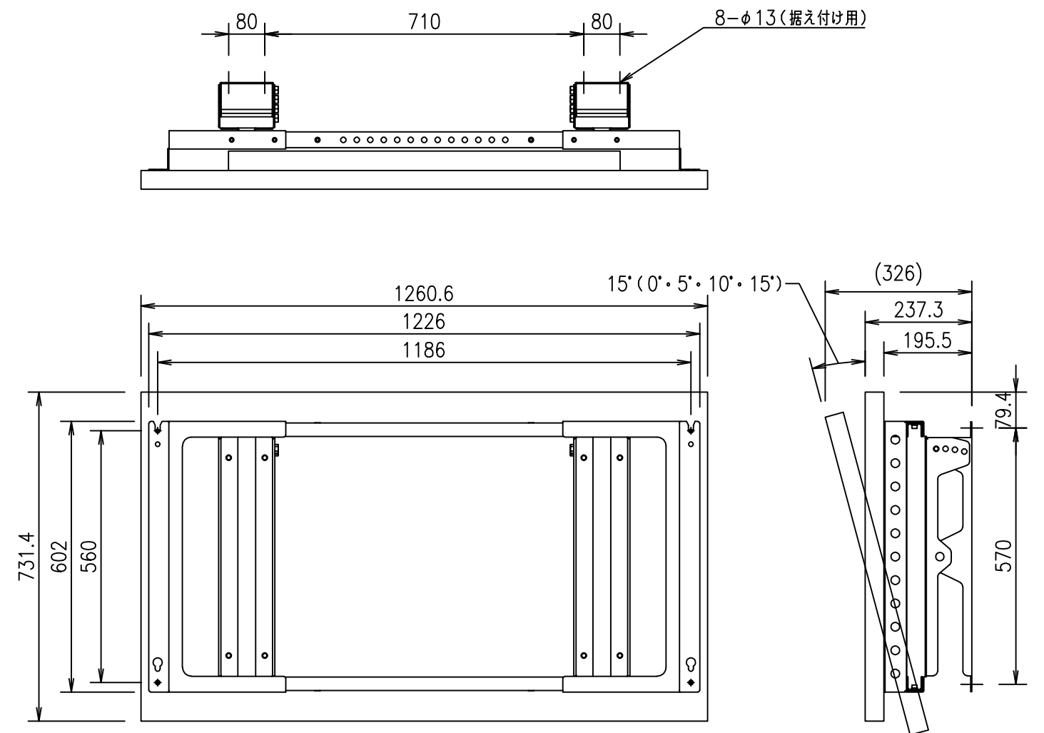
OH55 横向き設置
