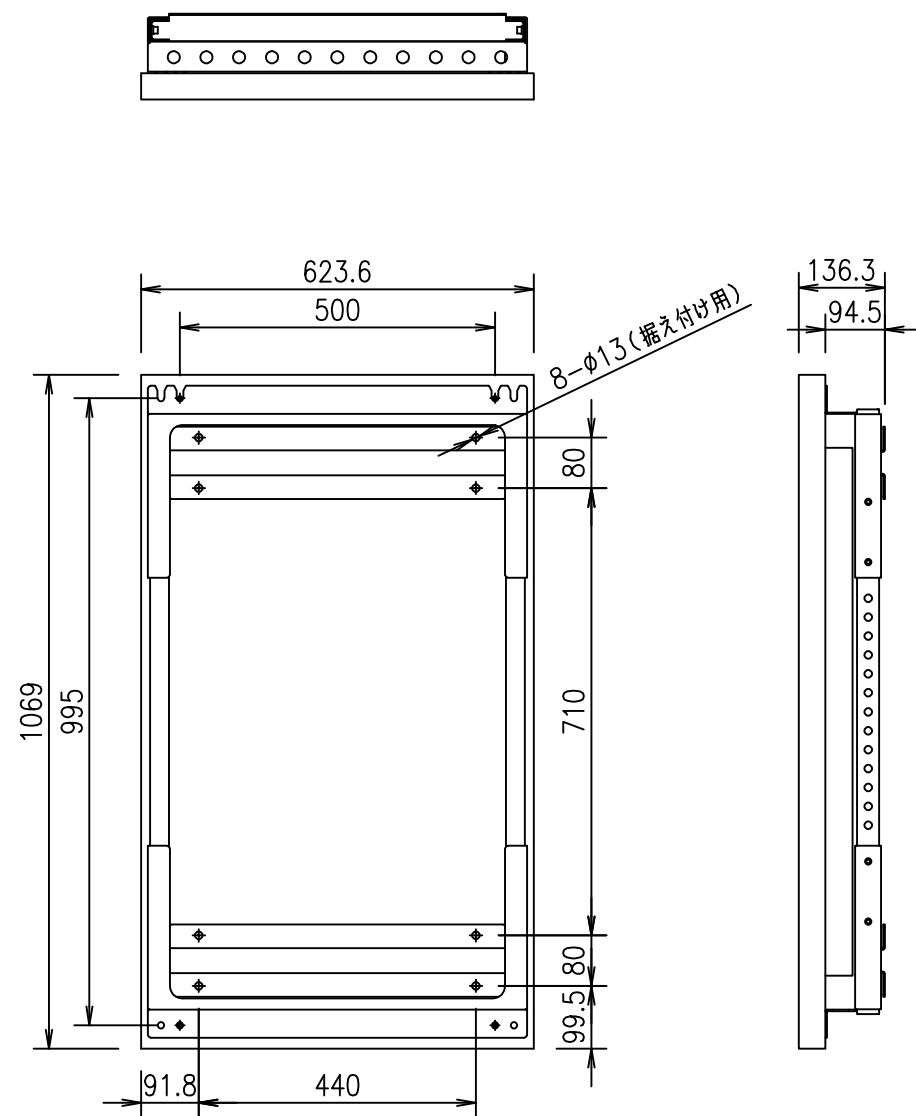
OH46 縦向き設置
