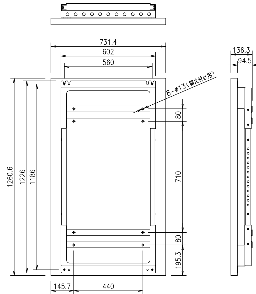
OH55 縦向き設置
