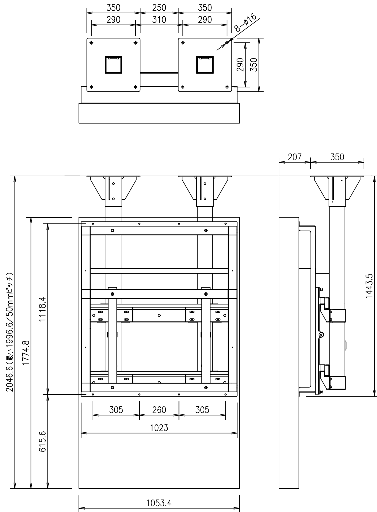
OH75 縦向き設置
