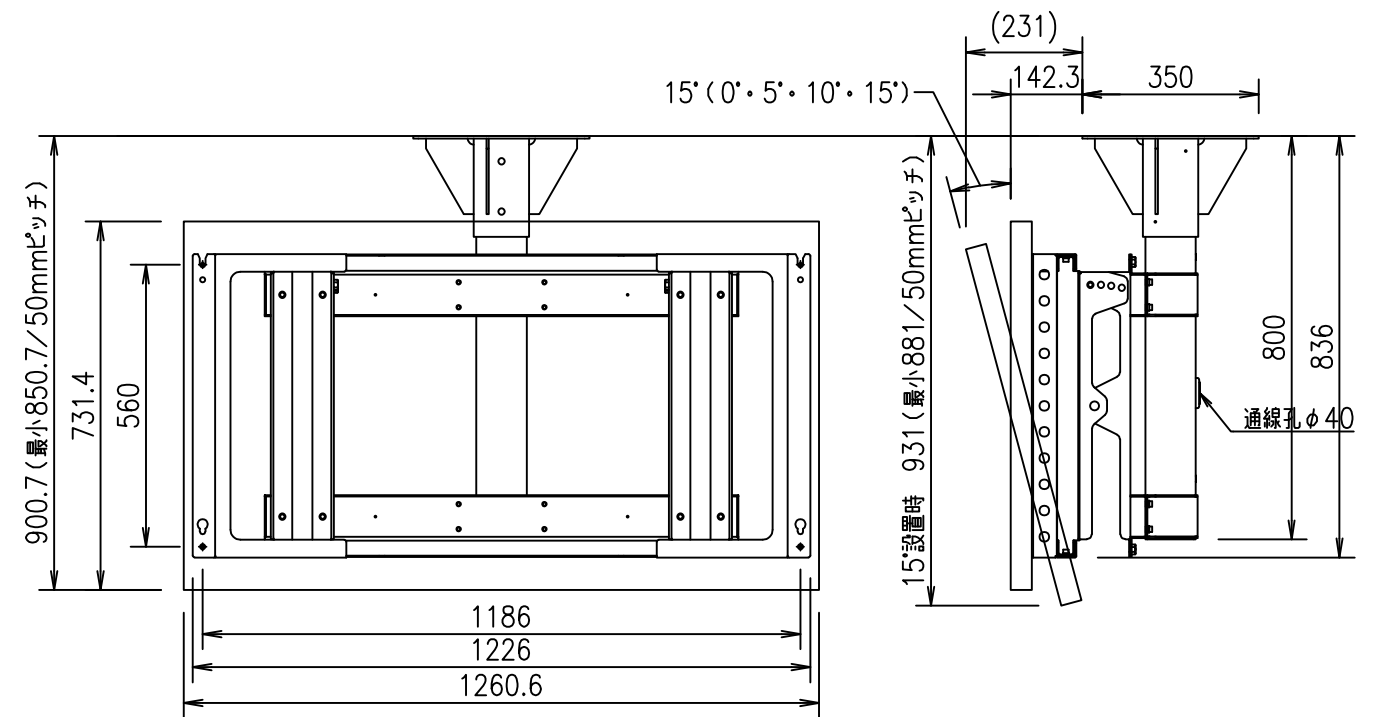
OH55 横向き設置
