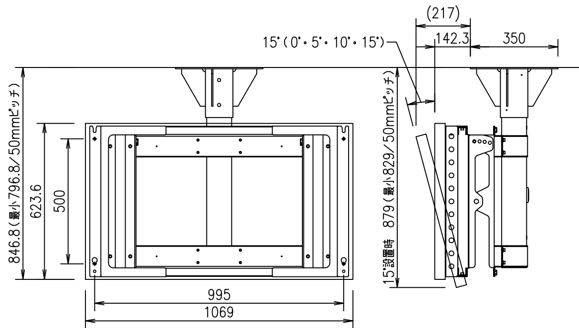
OH46 横向き設置
