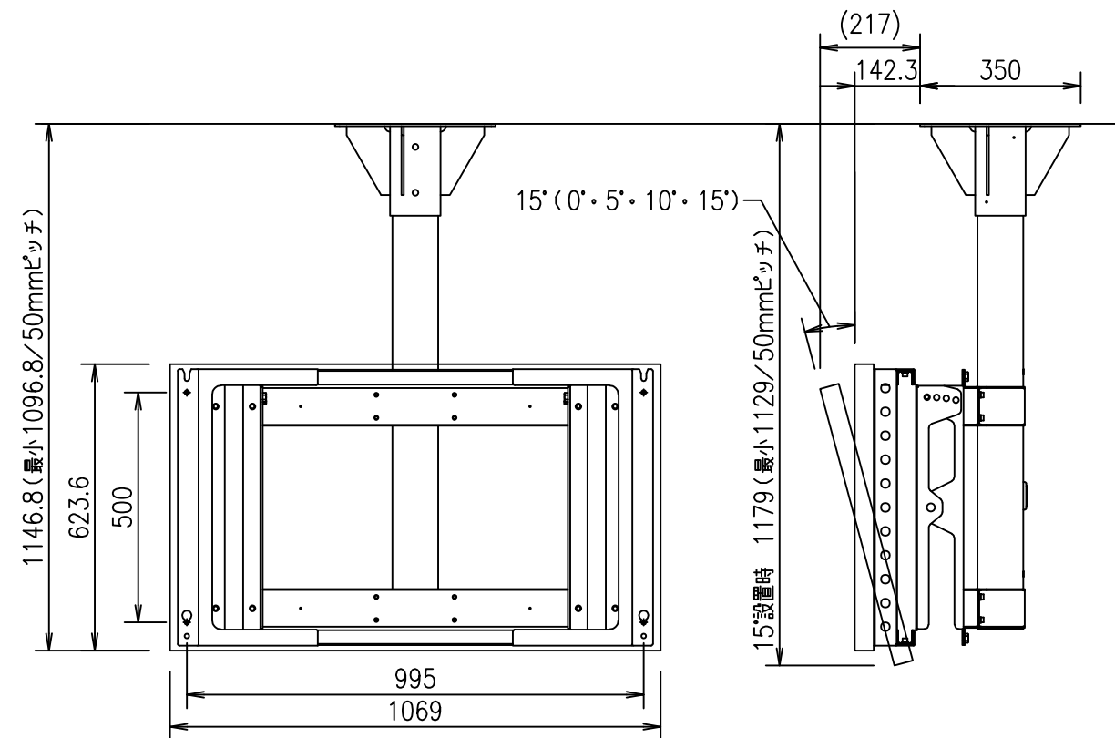
OH46 横向き設置
