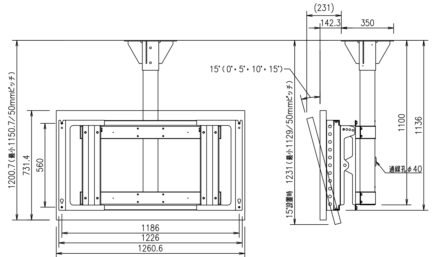
OH55 横向き設置
