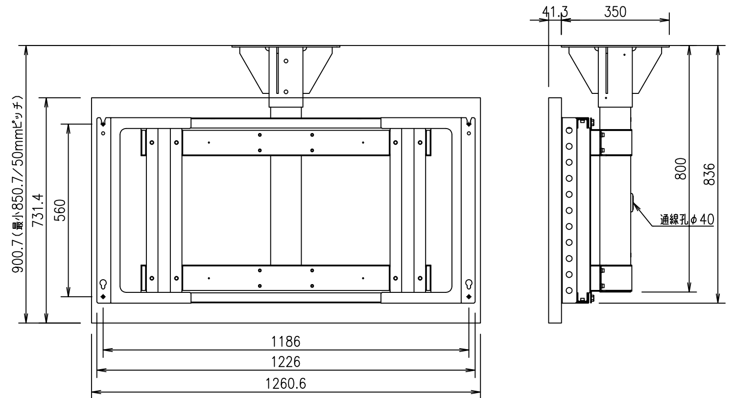
OH55 横向き設置
