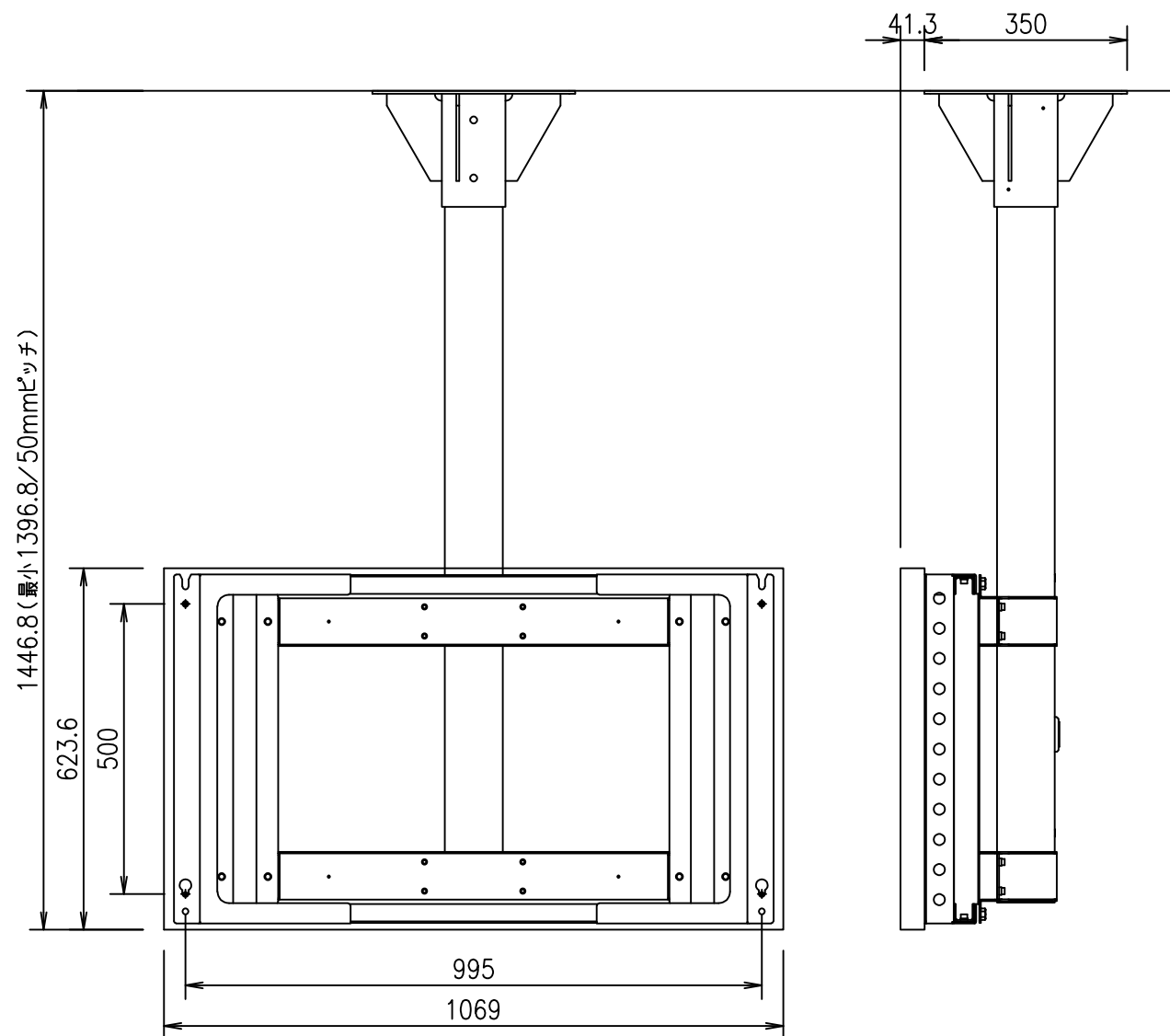
OH46 横向き設置
