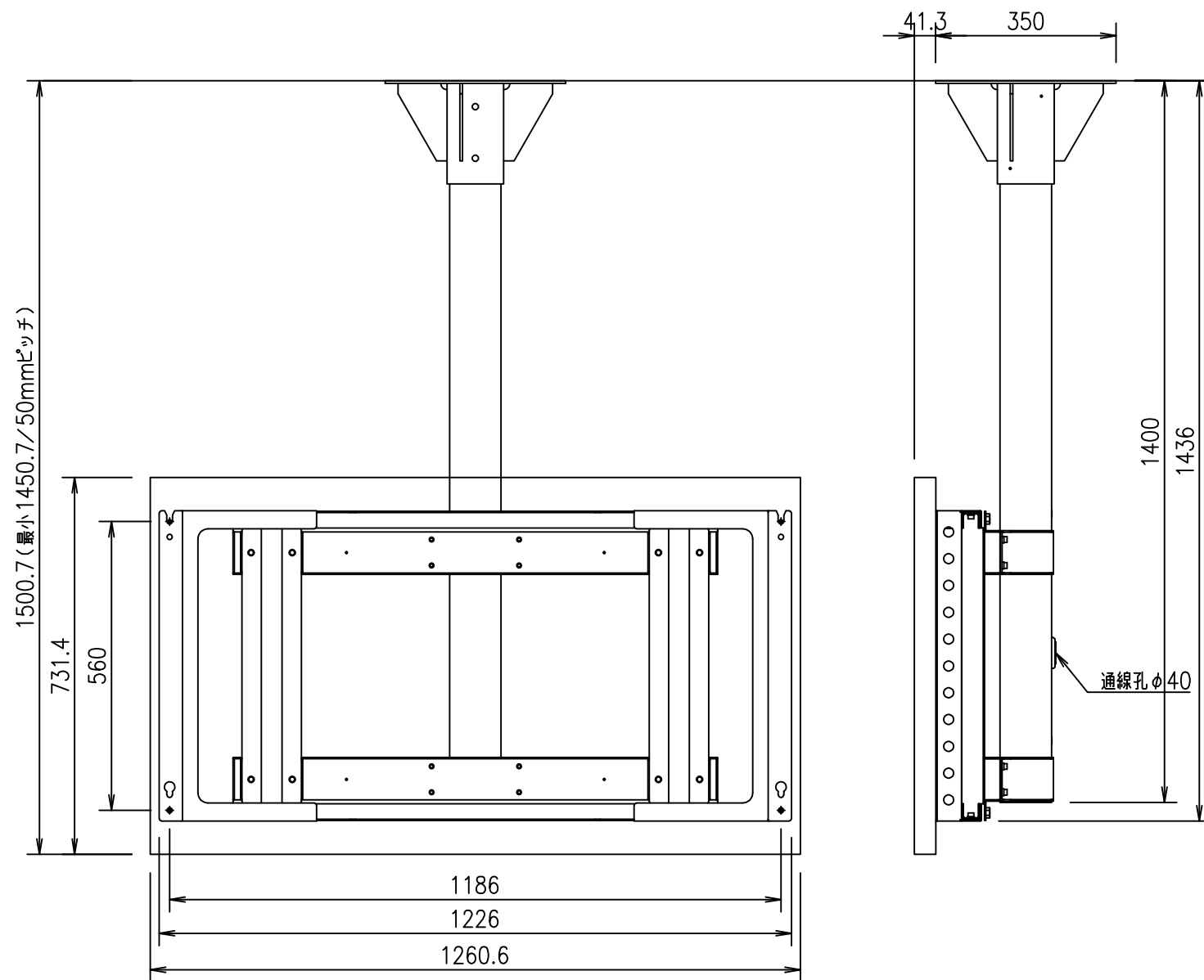
OH55 横向き設置
