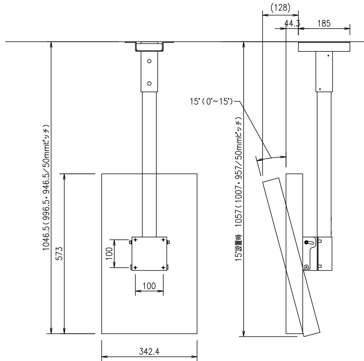
OH24 縦向き設置
