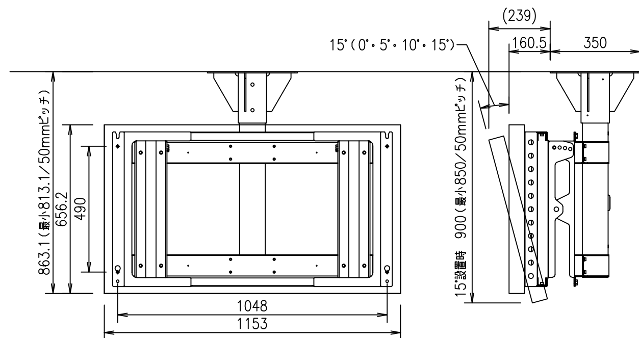
49XE3P-B 横向き設置
