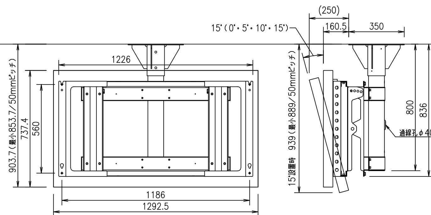
55XE3P-B 横向き設置
