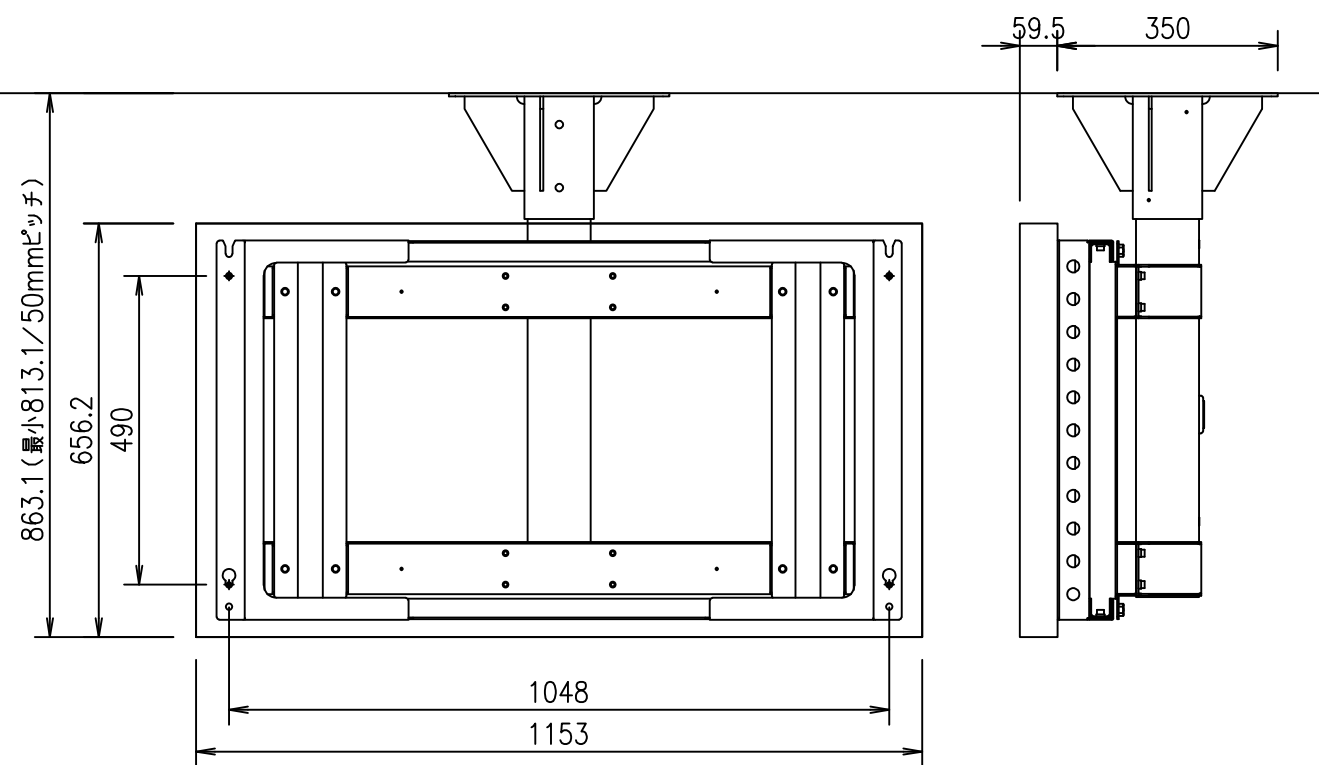
49XE3P-B 横向き設置
