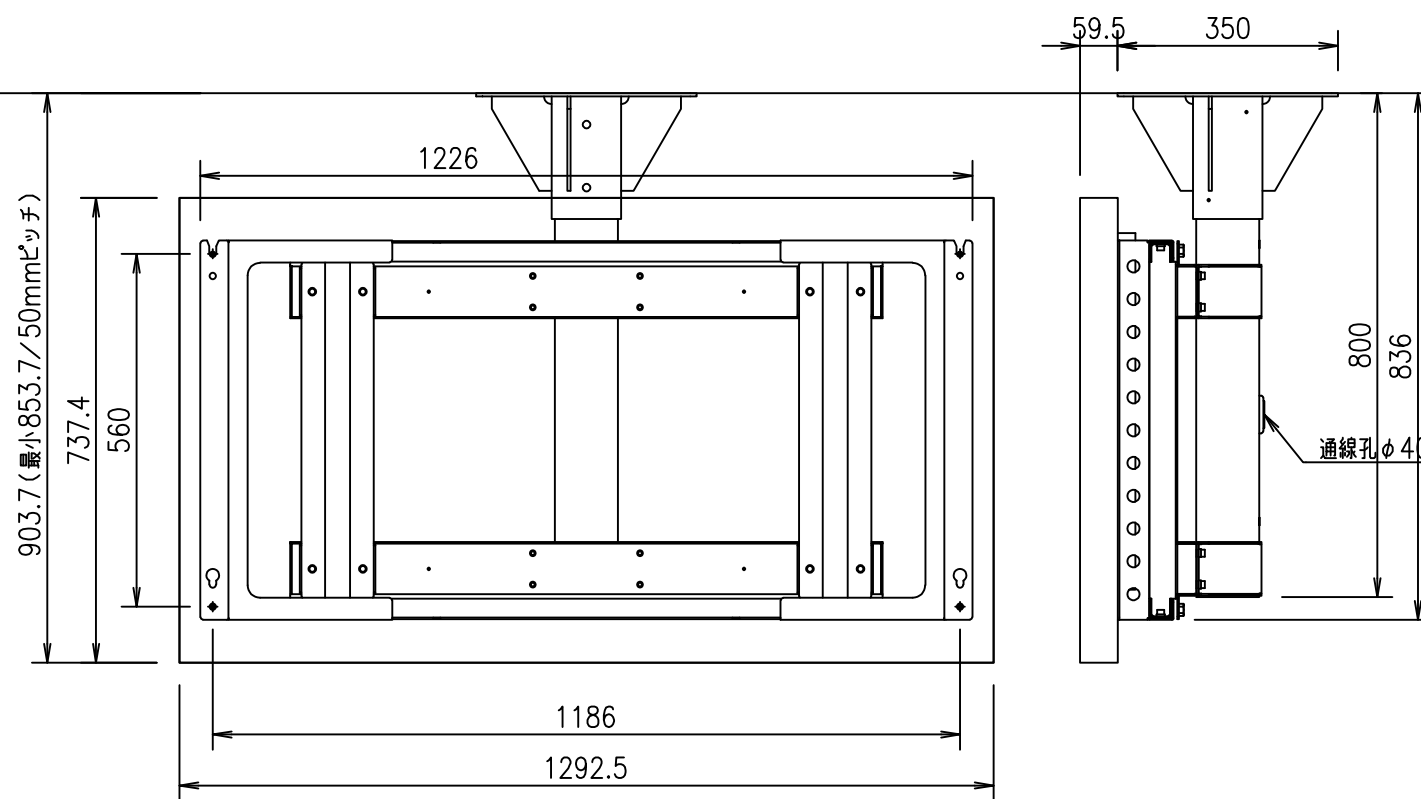
55XE3P-B 横向き設置
