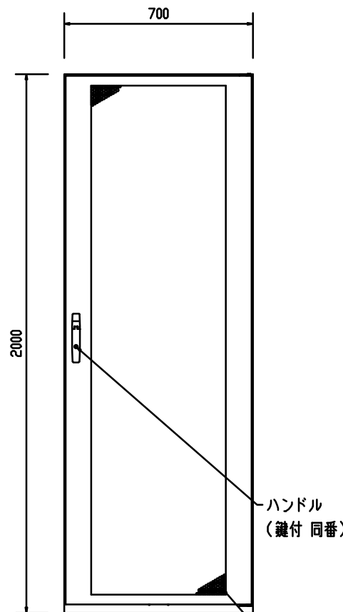
背面図
