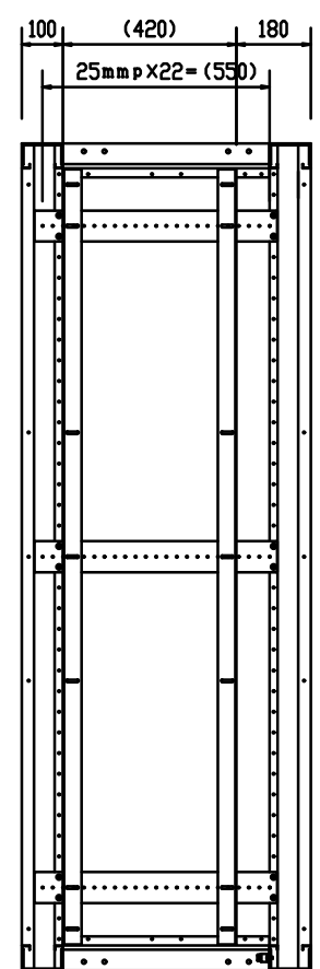
側面断面図
