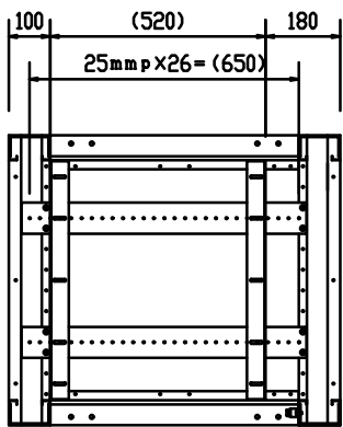
側面断面図
