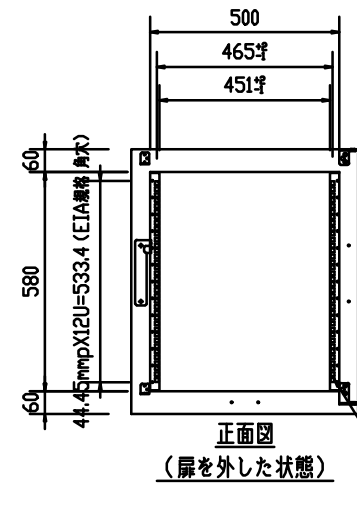
正面図 (扉を外した状態) マウントアングル (EIA規格 ケージナット仕様) (U表示付)
