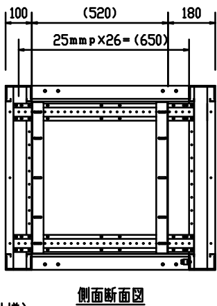
側面断面図
