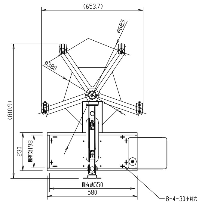
A-A 矢視図
