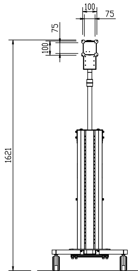
正面図
