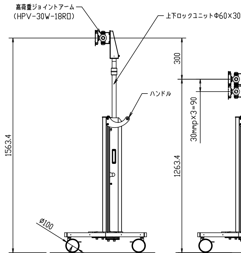
側面図 最高位置
