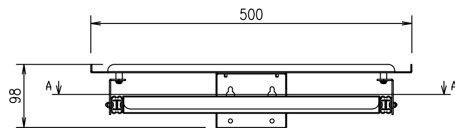
正面図
