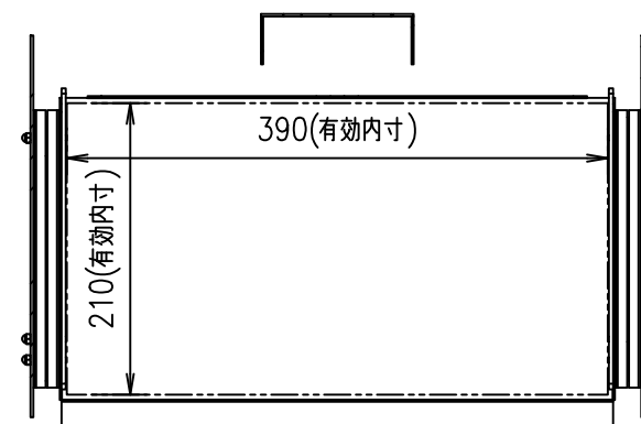
断面図A-A
