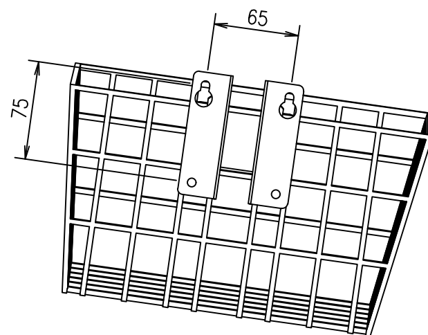
矢視図 A
