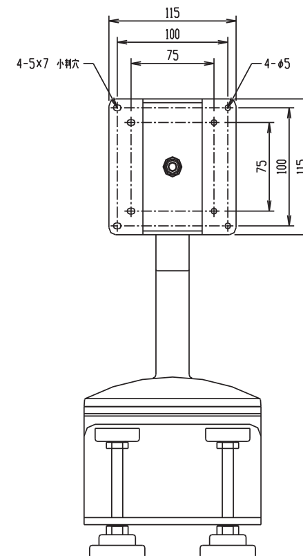
バルーンアーム2 標準タイプ本体+クランプ(大) FFP-BA75-BCB-2
