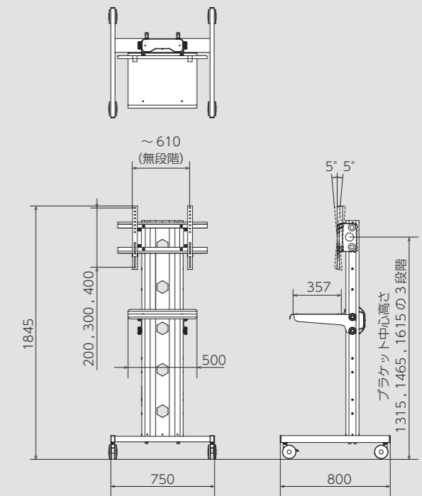
■寸法図
