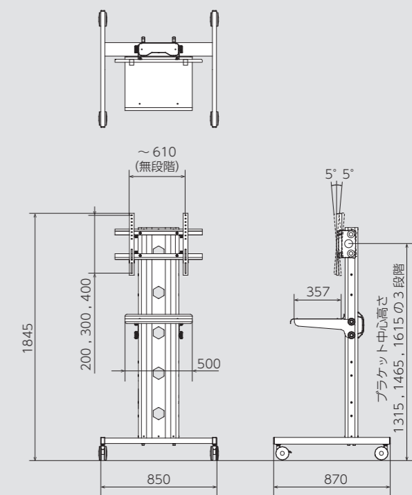
■寸法図
