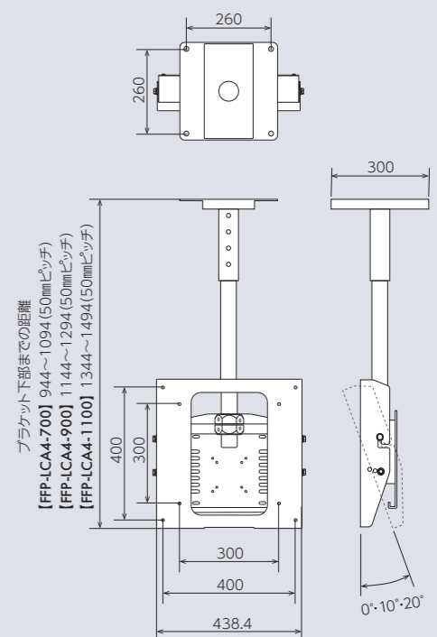
■寸法図
