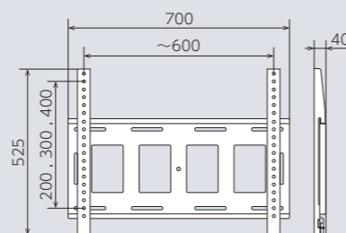
■寸法図
