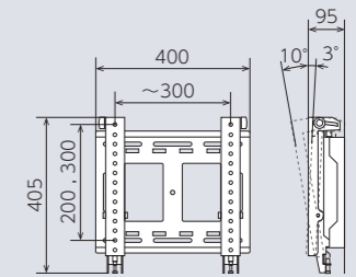
■寸法図
