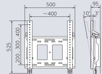
■寸法図
