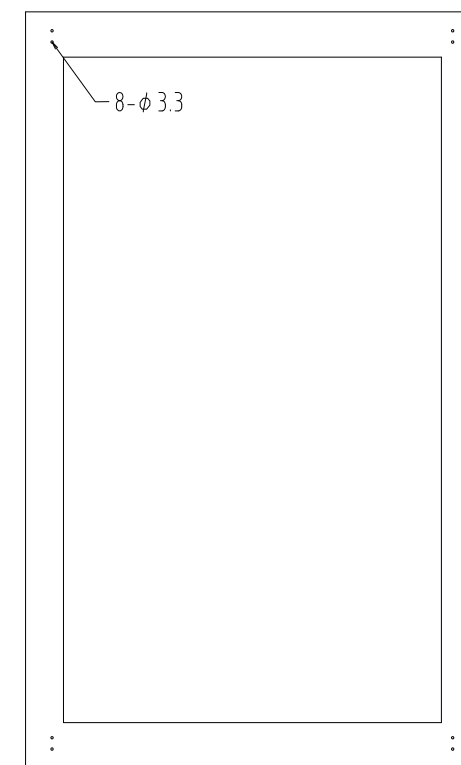
フレーム折戸用追加加工
