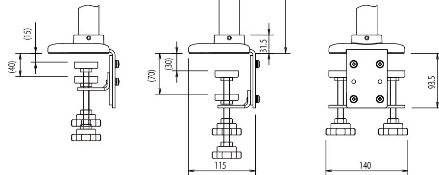
クレーン-ム-本体-デスククランプ-簡易ロック有り(型番:FFP-QAL-DC)
