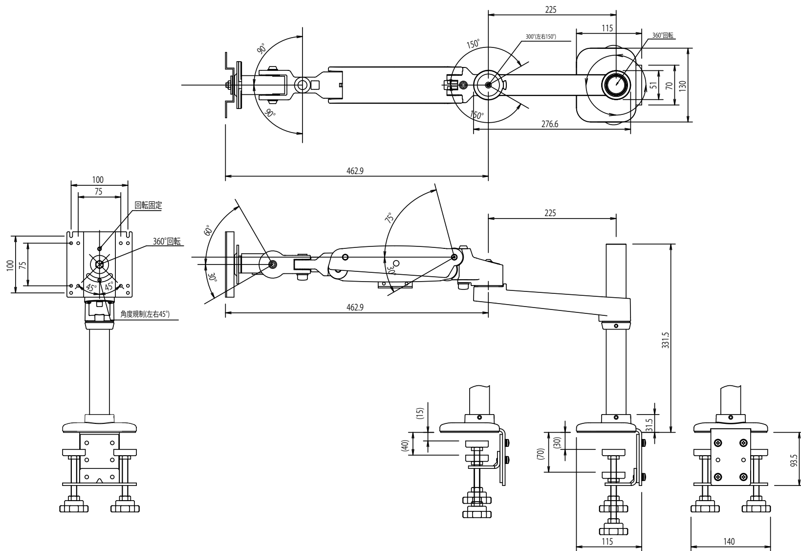
クレーン-ム-本体-デスククランプ-延長アーム-簡易ロック無し(型番:FFP-QA-DC-EF)
