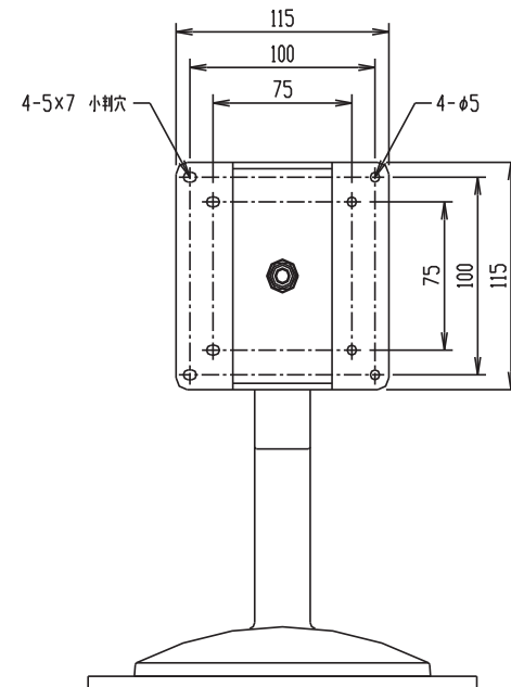
バルーンアーム2 高荷重タイプ本体 + 直付水平ベース (大) FFP-HBA75-BPB-2
