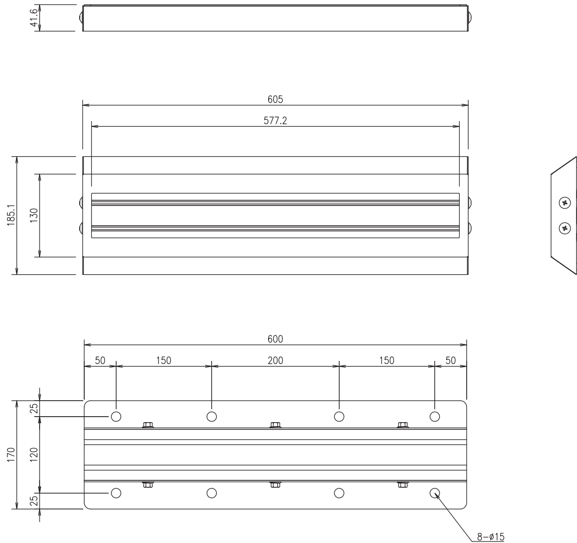
垂直面用アルミレール縦横兼用設置L600mmタイプ(型番:FTK-XYA600)
