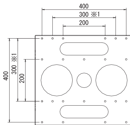
固定穴位置 (ディスプレイブラケット正面図)
