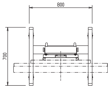
上面図
