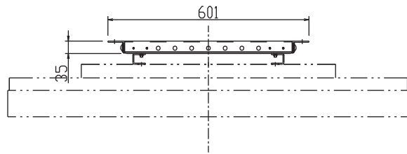
上面図
