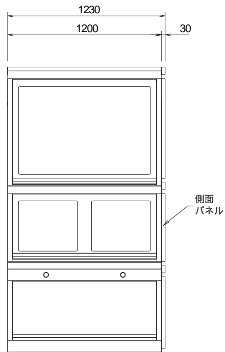
正面図 側面パネル有り(片側)
