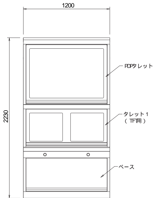
正面図 側面パネル無し
