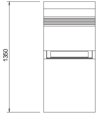
上面図 側面パネル無し
