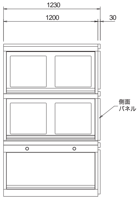
正面図 側面パネル有り(片側)
