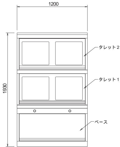
正面図 側面パネル無し
