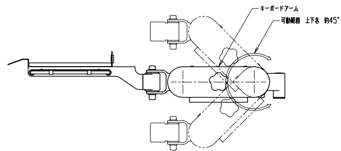
キーボードアーム可動範囲
