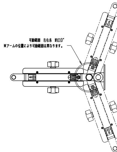
キーボードアーム可動範囲
