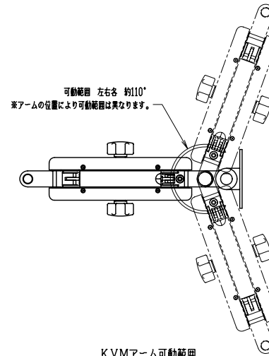
KVMアーム可動範囲
