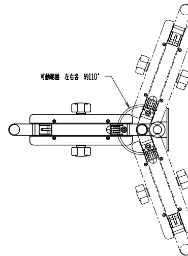
モニターアーム可動範囲
