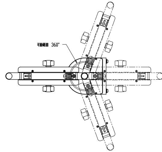
モニターアーム可動範囲
